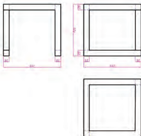
شکل ۸- سه نمای میز جلوی مبل
