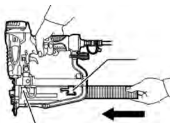
شکل ۱۰۲- بارگذاری منگنه
