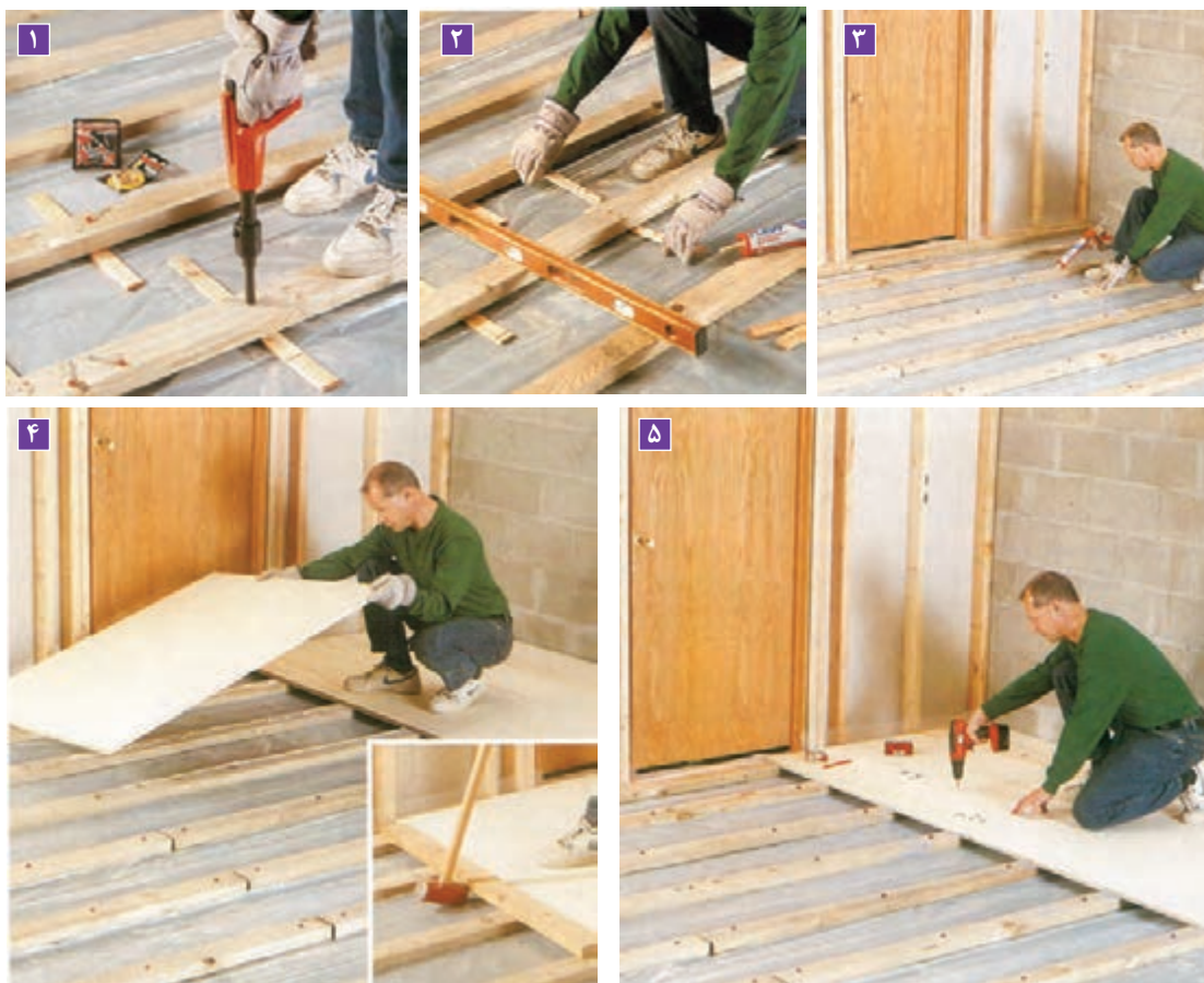
شکل ۴- مراحل نصب کف با تخته چوبی
