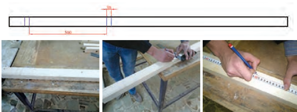
شکل ۴۱- اندازه‌گذاری و خط کشی محل قید افقی دوم
