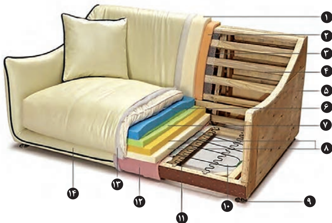
شکل ۵- مبیل راحتی و برشی از مواد به کار رفته در آن
