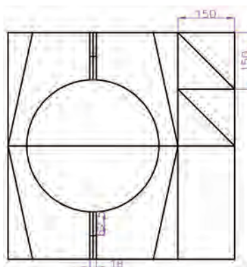
شکل ۳۹- خط‌کشی نبشی‌ها
