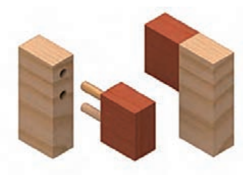
شکل ۲۶- اتصال دوبل
