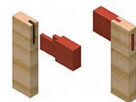
شکل ۲۵- اتصال کام و زبانه
